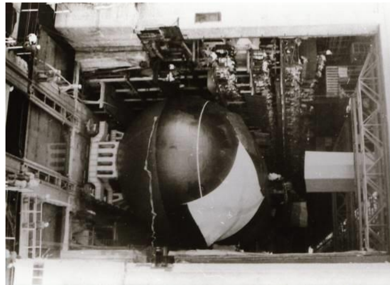
42. Фотонегатив. Коробков В.В. Вывод атомохода «ЩБ», проект 971 со ступеней Амурского судостроительного завода. 15.07.1994 Фотопленка черно-белая, негатив. 3,5х4 см. КП НВФ-9665/24
