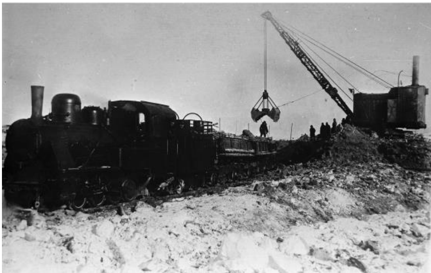
7. Фотонегатив сюжетный. Лоскутников А.Н. Копия с фотографии "Разработка котлована под строительство доков АСЗ. 1933 г." 1984 г. Фотопленка черно-белая, негатив черно-белый, копия с фотографии. 6х6 см. Пост. в 24.04.1984 г. Дар КП ОФ-8270/19
