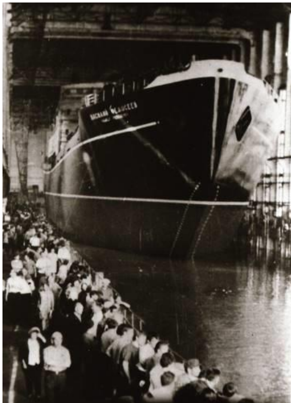
45. Фотонегатив. Коробков В.В. Вывод ледокольно-транспортного дизель-электрохода «Василий Федосеев». 1969 г. Фотопленка черно-белая, негатив. 3,5х4 см. КП НВФ-9677/2
